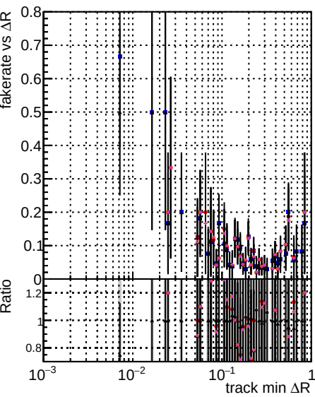
Fake rate vs \Delta R(\text{track, jet}) DQM mkFit5 XMinisNOPI base RetrainOldFiles125 v2 prelimWPM epoch4 RetrainOldFiles125 v2 ANDLessRetrain epoch4
