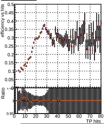
Efficiency vs hit Legend: DQM_mkFit5_XiMinusNOPU_base DQM_mkFit5_XiMinusNOPU_retrainOldFiles125_v2_prelimWPM_epoch4 DQM_mkFit6_XiMinusNOPU_base DQM_mkFit6_XiMinusNOPU_retrainOldFiles125_v2_prelimWPM_epoch4
