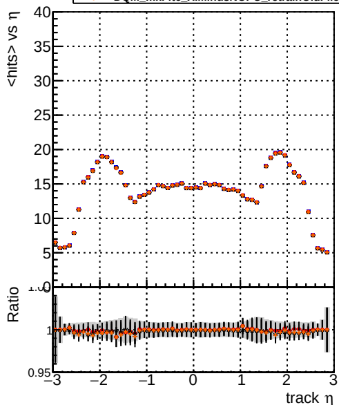
mean hits DQM_mkFit5_XiMinusNOPU_base DQM_mkFit5_XiMinusNOPU_retrainOldFiles125_v2_prelimWPM_epoch4 DQM_mkFit6_XiMinusNOPU_base DQM_mkFit6_XiMinusNOPU_retrainOldFiles125_v2_prelimWPM_epoch4
