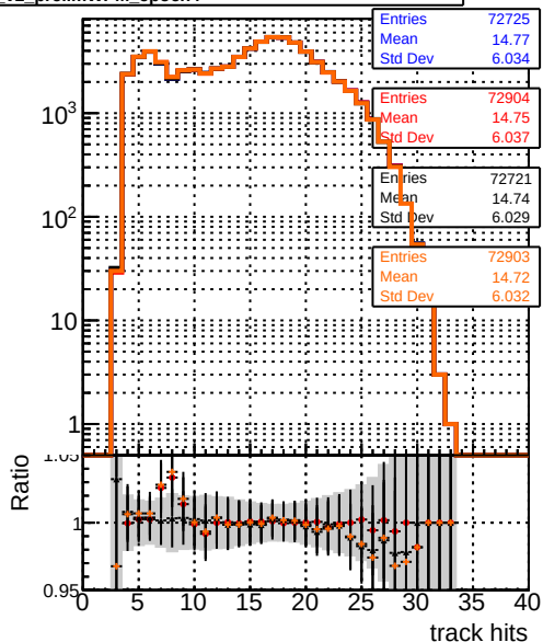
mean hits DQM_mkFit5_XiMinusNOPU_base DQM_mkFit5_XiMinusNOPU_retrainOldFiles125_v2_prelimWPM_epoch4 DQM_mkFit6_XiMinusNOPU_base DQM_mkFit6_XiMinusNOPU_retrainOldFiles125_v2_prelimWPM_epoch4
