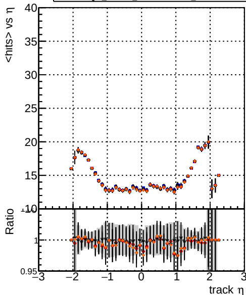
mean hits DQM_mkFit5_XiMinusNOPU_base DQM_mkFit5_XiMinusNOPU_retrainOldFiles125_v2_prelimWPM_epoch4 DQM_mkFit6_XiMinusNOPU_base DQM_mkFit6_XiMinusNOPU_retrainOldFiles125_v2_prelimWPM_epoch4
