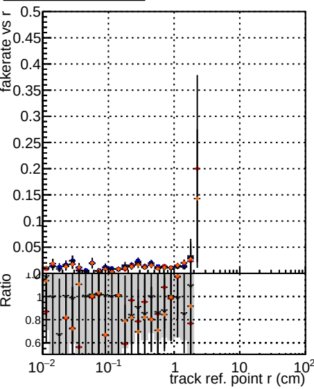
Fake rate vs vertpos base trainOldFiles125 v2 prelimWPM epoch4 base trainOldFiles125 v2 prelimWPM epoch4
