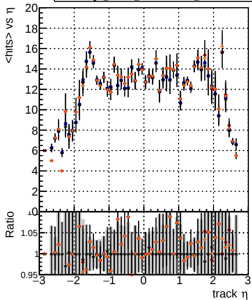
mean hit DQM_mkFit5_XiMinusNOPU_base DQM_mkFit5_XiMinusNOPU_retrainOldFiles125_v2_prelimWPM_epoch4 DQM_mkFit6_XiMinusNOPU_base DQM_mkFit6_XiMinusNOPU_retrainOldFiles125_v2_prelimWPM_epoch4
