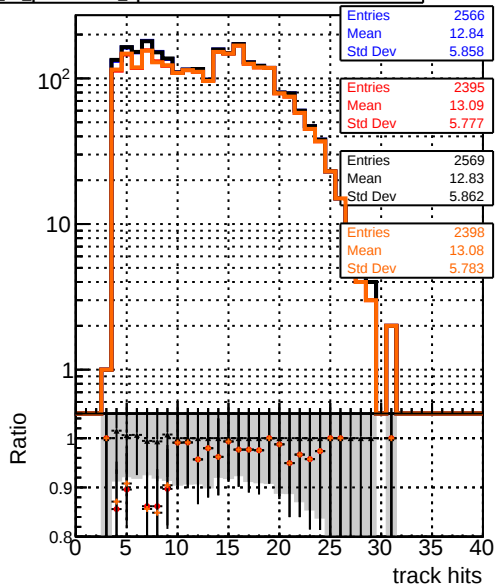
mean hit DQM_mkFit5_XiMinusNOPU_base DQM_mkFit5_XiMinusNOPU_retrainOldFiles125_v2_prelimWPM_epoch4 DQM_mkFit6_XiMinusNOPU_base DQM_mkFit6_XiMinusNOPU_retrainOldFiles125_v2_prelimWPM_epoch4
