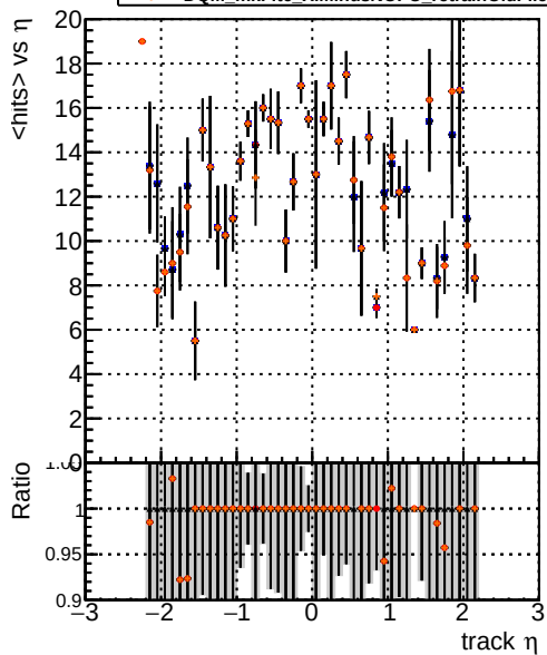
mean hit DQM_mkFit5_XiMinusNOPU_base DQM_mkFit5_XiMinusNOPU_retrainOldFiles125_v2_prelimWPM_epoch4 DQM_mkFit6_XiMinusNOPU_base DQM_mkFit6_XiMinusNOPU_retrainOldFiles125_v2_prelimWPM_epoch4
