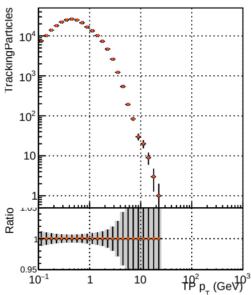
● DQM_mkFit5_XiMinusNOPU_base ◆ DQM_mkFit5_XiMinusNOPU_retrainOldFiles125_v2_prelimWPM_epoch4 ▲ DQM_mkFit6_XiMinusNOPU_base ★ DQM_mkFit6_XiMinusNOPU_retrainOldFiles125_v2_prelimWPM_epoch4
