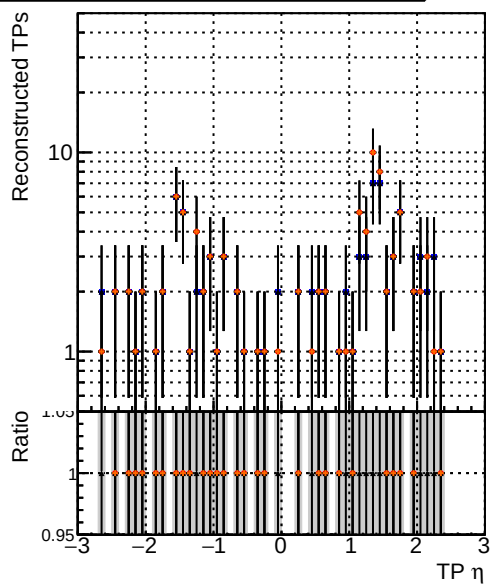
● DQM_mkFit5_XiMinusNOPU_base ◆ DQM_mkFit5_XiMinusNOPU_retrainOldFiles125_v2_prelimWPM_epoch4 ▲ DQM_mkFit6_XiMinusNOPU_base ★ DQM_mkFit6_XiMinusNOPU_retrainOldFiles125_v2_prelimWPM_epoch4
