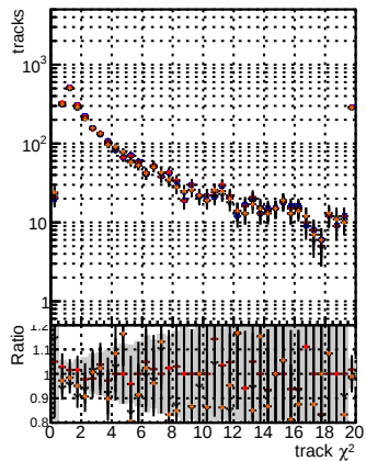
N of reco track vs. s DQM mkrE15 XIMinusNOPU base DQM mkrE15 XIMinusNOPU base DQM mkrE16 XIMinusNOPU base retrainOldFiles125_v2_prelimWPM_epoch4
