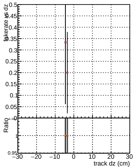
DOM mkrf15 X M H N O P U base trainOldFiles125 v2 prelimWPM epoch4 DOM mkrf16 X M H N O P U base trainOldFiles125 v2 prelimWPM epoch4 Fake rate vs d
