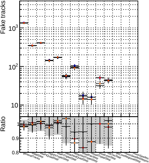
Number Model 1 DQM_mkFit6_XiMinusNOPU_base 2 DQM_mkFit6_XiMinusNOPU_retrainOldFiles125_v2_prelimWPM_epoch4
