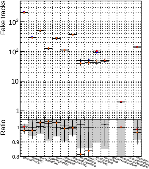
Number — DQM_mkFit6_XiMinusNOPU_base — DQM_mkFit6_XiMinusNOPU_retrainOldFiles125_v2_prelimWPM_epoch4
