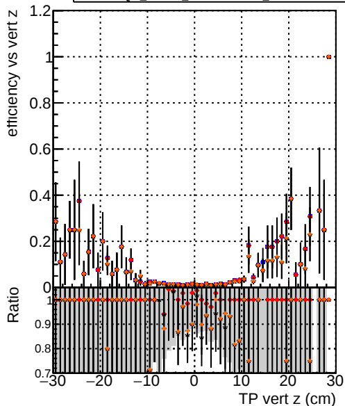
Efficiency vs vert z —●— DQM_mkFit5_XiMinusNOPU_base —●— DQM_mkFit5_XiMinusNOPU_retrainOldFiles125_v2_prelimWPM_epoch4 —●— DQM_mkFit6_XiMinusNOPU_base —●— DQM_mkFit6_XiMinusNOPU_retrainOldFiles125_v2_prelimWPM_epoch4
