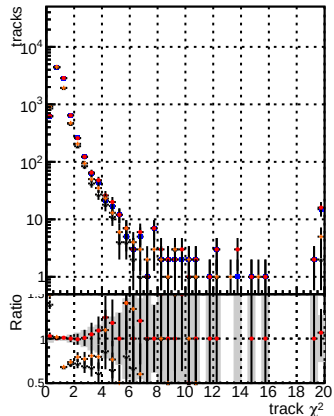
N of reco track vs. \chi^2 BSM M1E15 M1E16 M1E17 M1E18 M1E19 M1E20 M1E21 M1E22 M1E23 M1E24 M1E25 M1E26 M1E27 M1E28 M1E29 M1E30 M1E31 M1E32 M1E33 M1E34 M1E35 M1E36 M1E37 M1E38 M1E39 M1E40
