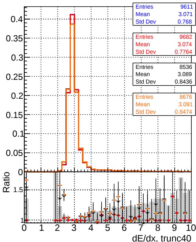
dE/dx estimator 2
