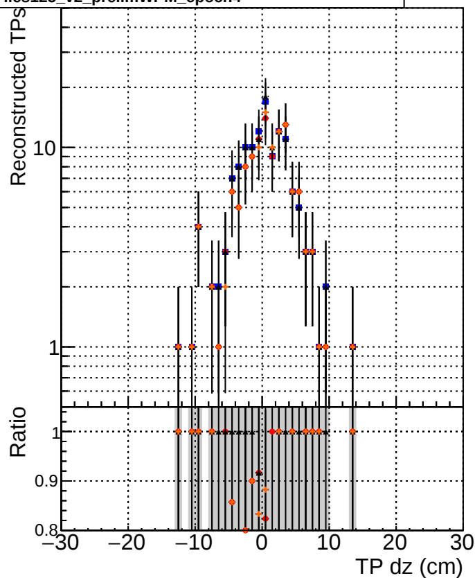
DQM_mkFit5_XiMinusPU_base DQM_mkFit5_XiMinusPU_retrainOldFiles125_v2_prelimWPM_epoch4 DQM_mkFit6_XiMinusPU_base DQM_mkFit6_XiMinusPU_retrainOldFiles125_v2_prelimWPM_epoch4
