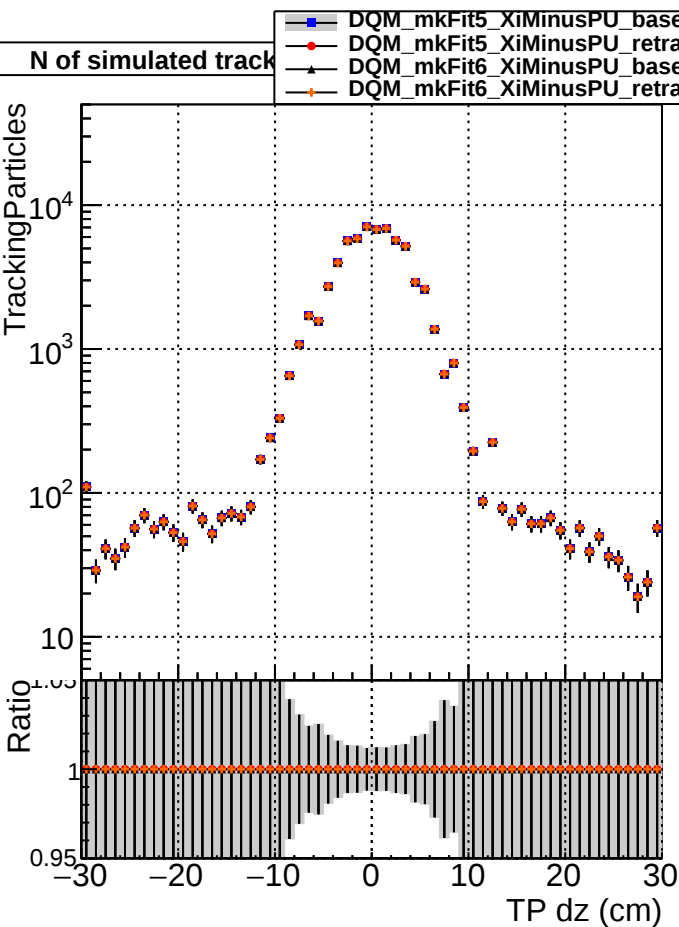
DQM_mkFit5_XiMinusPU_base DQM_mkFit5_XiMinusPU_retrainOldFiles125_v2_prelimWPM_epoch4 DQM_mkFit6_XiMinusPU_base DQM_mkFit6_XiMinusPU_retrainOldFiles125_v2_prelimWPM_epoch4
