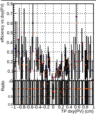
Efficiency vs Dxy(PV) Legend: DQM_mkFit5_XiMinusPU_base DQM_mkFit5_XiMinusPU_retrainOldFiles125_v2_prelimWPM_epoch4 DQM_mkFit6_XiMinusPU_base DQM_mkFit6_XiMinusPU_retrainOldFiles125_v2_prelimWPM_epoch4
