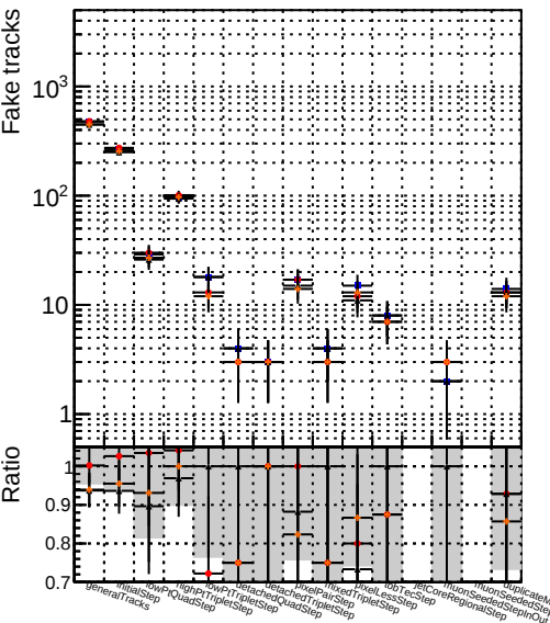
Number Model 1 DQM mkFit6_XiMinusPU_base 2 DQM mkFit6_XiMinusPU_retrainOldFiles125_v2_prelimWPM_epoch4
