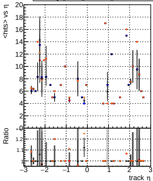
mean hit — DQM_mkFit5_XiMinusPU_base — DQM_mkFit5_XiMinusPU_retrainOldFiles125_v2_prelimWPM_epoch4 — DQM_mkFit6_XiMinusPU_base — DQM_mkFit6_XiMinusPU_retrainOldFiles125_v2_prelimWPM_epoch4
