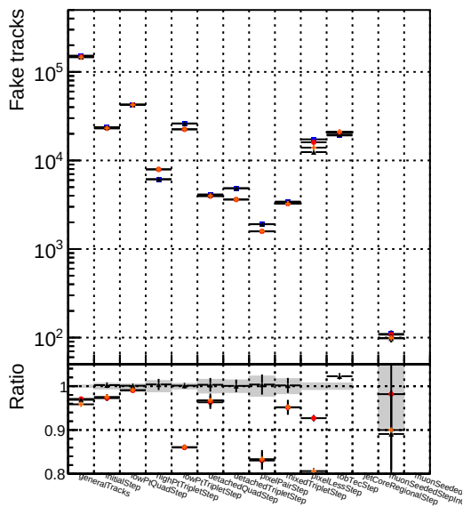
Number Model 1 DQM mkFit6 XiMinusPU base 2 DQM mkFit6 XiMinusPU retrainOldFiles125 v2_prelimWPM_epoch4
