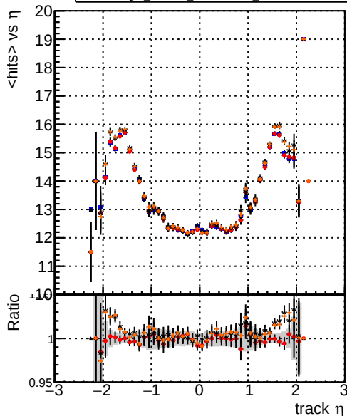
mean hits DQM_mkFit5_XiMinusPU_base DQM_mkFit5_XiMinusPU_retrainOldFiles125_v2_prelimWPM_epoch4 DQM_mkFit6_XiMinusPU_base DQM_mkFit6_XiMinusPU_retrainOldFiles125_v2_prelimWPM_epoch4
