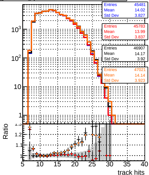
mean hits DQM_mkFit5_XiMinusPU_base DQM_mkFit5_XiMinusPU_retrainOldFiles125_v2_prelimWPM_epoch4 DQM_mkFit6_XiMinusPU_base DQM_mkFit6_XiMinusPU_retrainOldFiles125_v2_prelimWPM_epoch4
