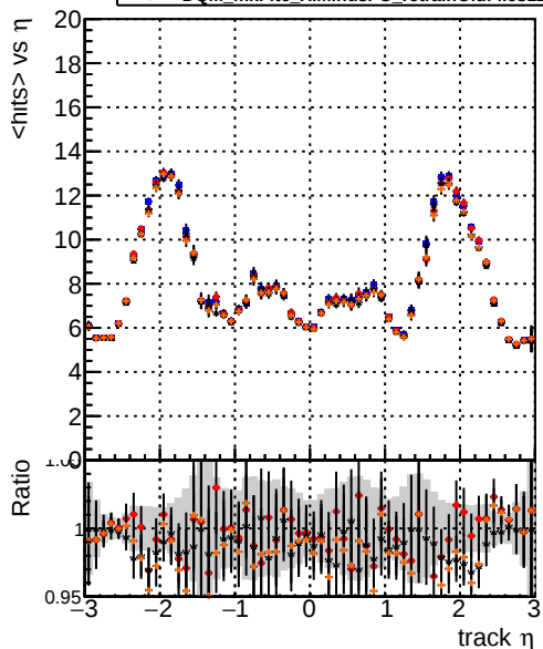
mean hits vs \eta DQM_mkFit5_XiMinusPU_base DQM_mkFit5_XiMinusPU_retrainOldFiles125_v2_prelimWPM_epoch4 DQM_mkFit6_XiMinusPU_base DQM_mkFit6_XiMinusPU_retrainOldFiles125_v2_prelimWPM_epoch4
