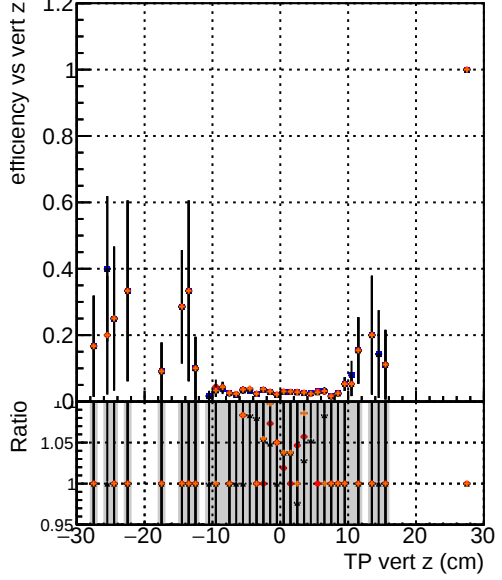
Efficiency vs vert z —•— DQM_mkFit5_XiMinusPU_base —•— DQM_mkFit5_XiMinusPU_retrainOldFiles125_v2_prelimWPM_epoch4 —•— DQM_mkFit6_XiMinusPU_base —•— DQM_mkFit6_XiMinusPU_retrainOldFiles125_v2_prelimWPM_epoch4
