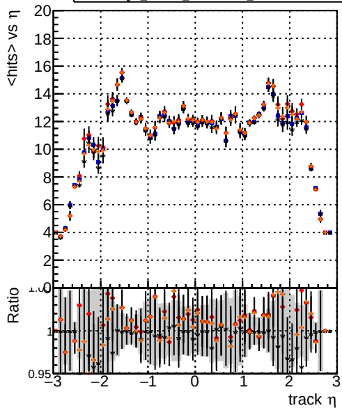
mean hits DQM_mkFit5_XiMinusPU_base DQM_mkFit5_XiMinusPU_retrainOldFiles125_v2_prelimWPM_epoch4 DQM_mkFit6_XiMinusPU_base DQM_mkFit6_XiMinusPU_retrainOldFiles125_v2_prelimWPM_epoch4
