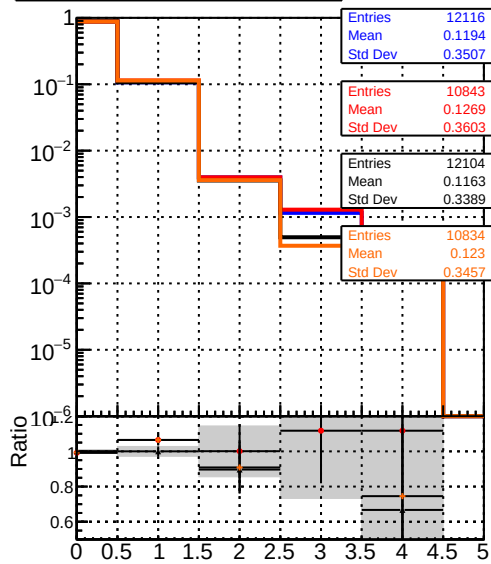
mean hits DQM_mkFit5_XiMinusPU_base DQM_mkFit5_XiMinusPU_retrainOldFiles125_v2_prelimWPM_epoch4 DQM_mkFit6_XiMinusPU_base DQM_mkFit6_XiMinusPU_retrainOldFiles125_v2_prelimWPM_epoch4
