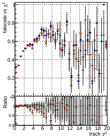
Fake rate vs. BQM mkFit5 XIM MIPUS BQM mkFit5 XIM MIPUS BQM mkFit5 XIM MIPUS BQM mkFit5 XIM MIPUS BQM mkFit5 XIM MIPUS BQM mkFit5 XIM MIPUS BQM mkFit5 XIM MIPUS BQM mkFit5 XIM MIPUS BQM mkFit5 XIM MIPUS BQM mkFit5 XIM MIPUS BQM mkFit5 XIM MIPUS BQM mkFit5 XIM MIPUS BQM mkFit5 XIM MIPUS BQM mkFit5 XIM MIPUS BQM mkFit5 XIM MIPUS BQM mkFit5 XIM MIPUS BQM mkFit5 XIM MIPUS BQM mkFit5 XIM MIPUS BQM mkFit5 XIM MIPUS BQM mkFit5 XIM MIPUS BQM mkFit5 XIM MIPUS BQM mkFit5 XIM MIPUS BQM mkFit5 XIM MIPUS BQM mkFit5 XIM MIPUS BQM mkFit5 XIM MIPUS BQM mkFit5 XIM MIPUS BQM mkFit5 XIM MIPUS BQM mkFit5 XIM MIPUS BQM mkFit5 XIM MIPUS BQM mkFit5 XIM MIPUS BQM mkFit5 XIM MIPUS BQM mkFit5 XIM MIPUS BQM mkFit5 XIM MIPUS BQM mkFit5 XIM MIPUS BQM mkFit5 XIM MIPUS BQM mkFit5 XIM MIPUS BQM mkFit5 XIM MIPUS BQM mkFit5 XIM MIPUS BQM mkFit5 XIM MIPUS BQM mkFit5 XIM MIPUS BQM mkFit5 XIM MIPUS BQM mkFit5 XIM MIPUS BQM mkFit5 XIM MIPUS BQM mkFit5 XIM MIPUS BQM mkFit5 XIM MIPUS BQM mkFit5 XIM MIPUS BQM mkFit5 XIM MIPUS BQM mkFit5 XIM MIPUS BQM mkFit5 XIM MIPUS BQM mkFit5 XIM MIPUS BQM mkFit5 XIM MIPUS BQM mkFit5 XIM MIPUS BQM mkFit5 XIM MIPUS BQM mkFit5 XIM MIPUS BQM mkFit5 XIM MIPUS BQM mkFit5 XIM MIPUS BQM mkFit5 XIM MIPUS BQM mkFit5 XIM MIPUS BQM mkFit5 XIM MIPUS BQM mkFit5 XIM MIPUS BQM mkFit5 XIM
