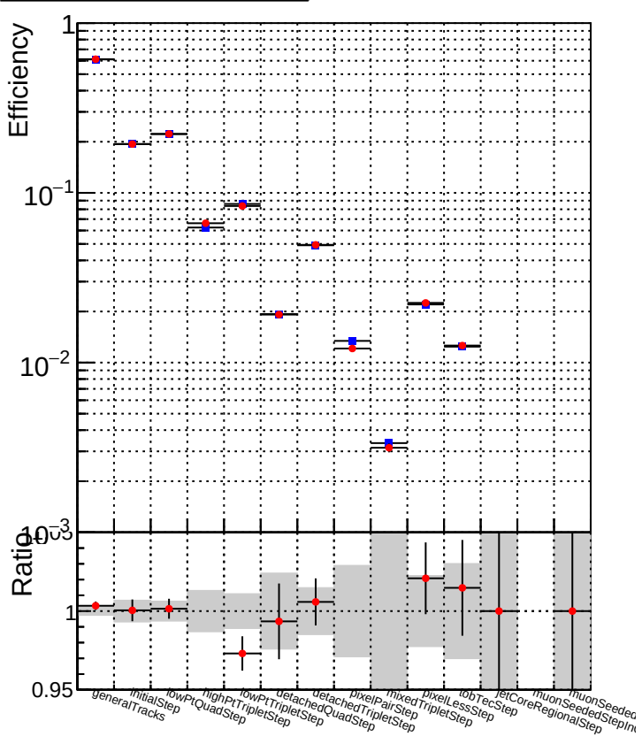
DQM_mkFit_TTbase DQM_mkFit5_TT_retrainOldFiles125_v2_prelimWP_epoch4
