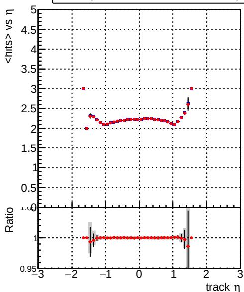
mean hits — DQM_mkFit_TTbase — DQM_mkFit5_TT_retrainOldFiles125_v2_prelimWP_epoch4
