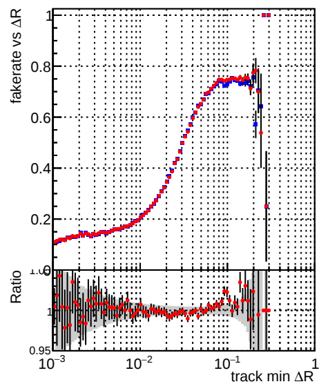
—•— DQM_mkFit_TTbase —•— DQM_mkFit5_TT_retrainOldFiles125_v2_prelimWP_epoch4
