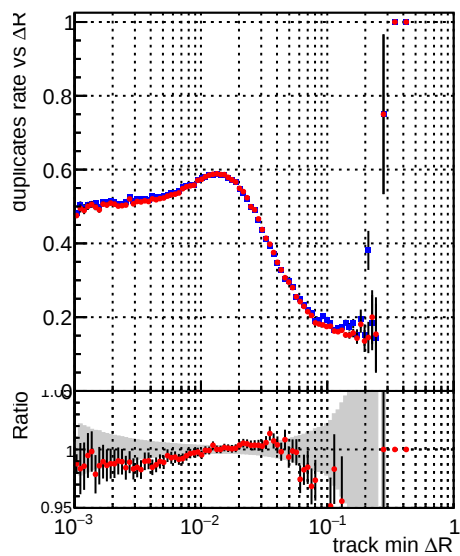
—•— DQM_mkFit_TTbase —•— DQM_mkFit5_TT_retrainOldFiles125_v2_prelimWP_epoch4
