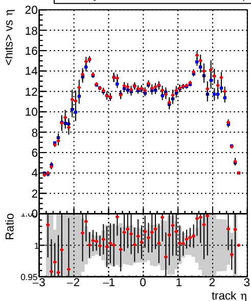
— DQM_mkFit_TTbase — DQM_mkFit5_TT_retrainOldFiles125_v2_prelimWP_epoch4
