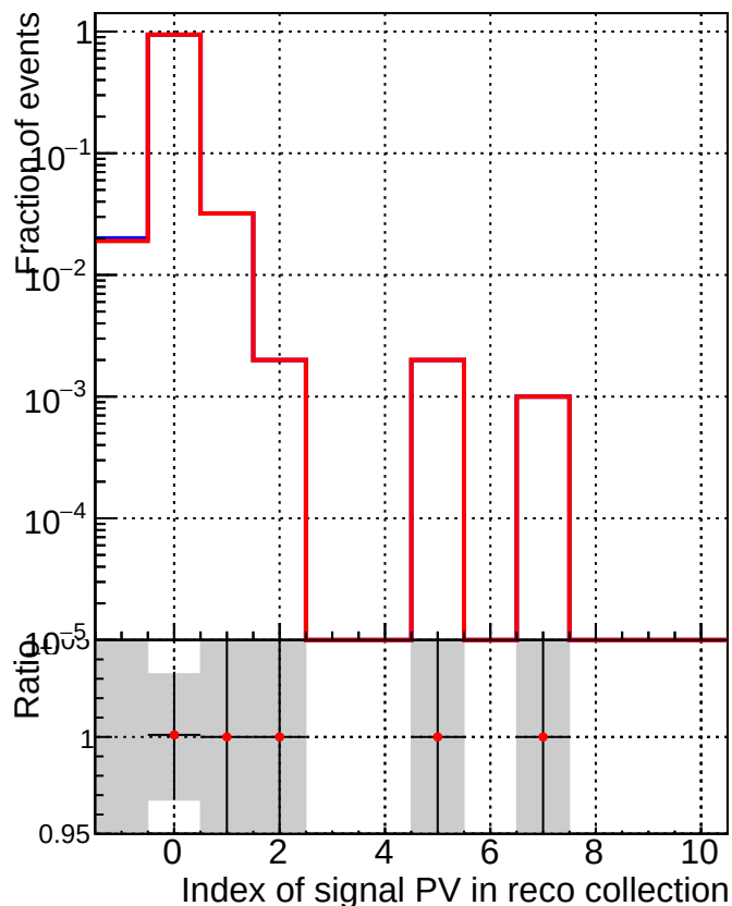
■ DQM_mkFit_TTbase ● DQM_mkFit5_TT_retrainOldFiles125_v2_prelimWP_epoch4
