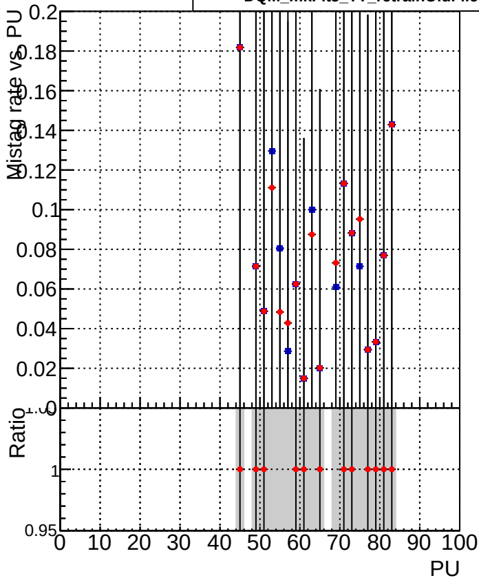
■ DQM_mkFit_TTbase ● DQM_mkFit5_TT_retrainOldFiles125_v2_prelimWP_epoch4
