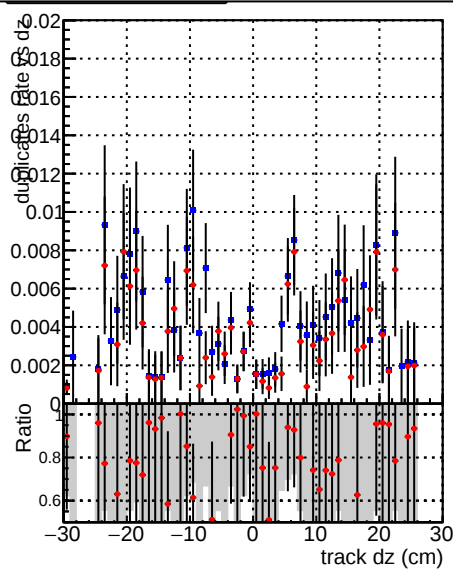
—●— DQM_mkFit_TTbase —●— DQM_mkFit5_TT_retrainOldFiles125_v2_prelimWP_epoch4
