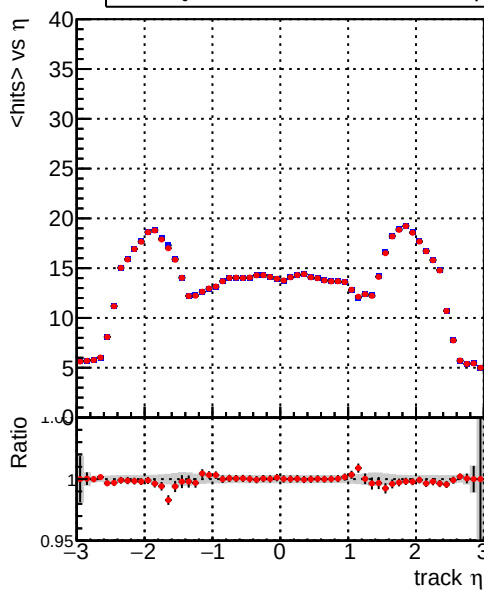
— DQM_mkFit5_TTbase — DQM_mkFit5_TT_retrainOldFiles125_v2_prelimWP_epoch4
