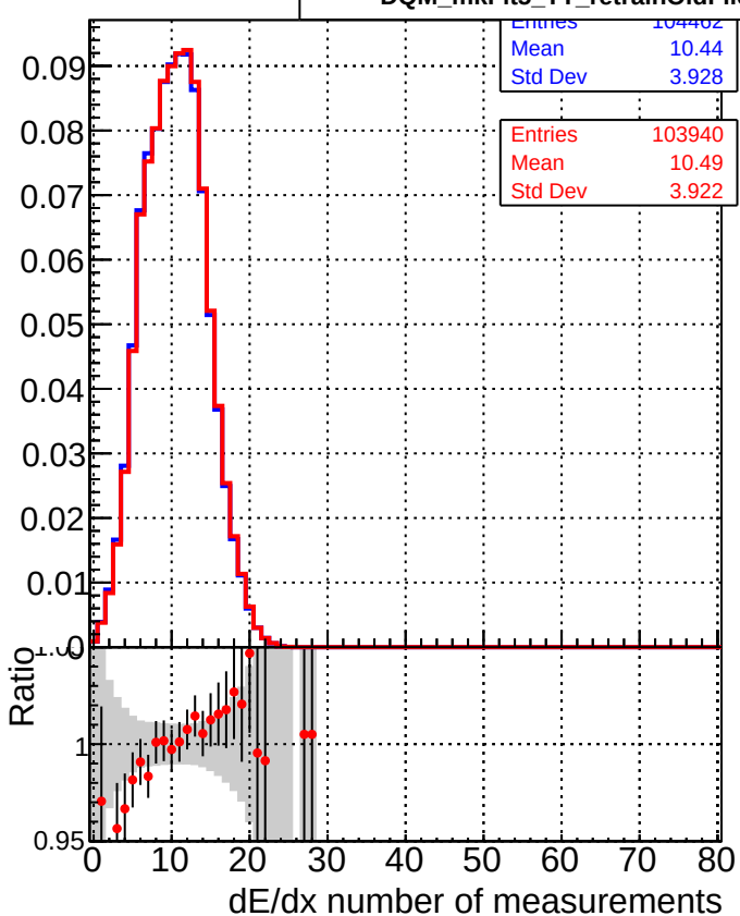
■ DQM_mkFit_TTbase ● DQM_mkFit5_TT_retrainOldFiles125_v2_prelimWP_epoch4
