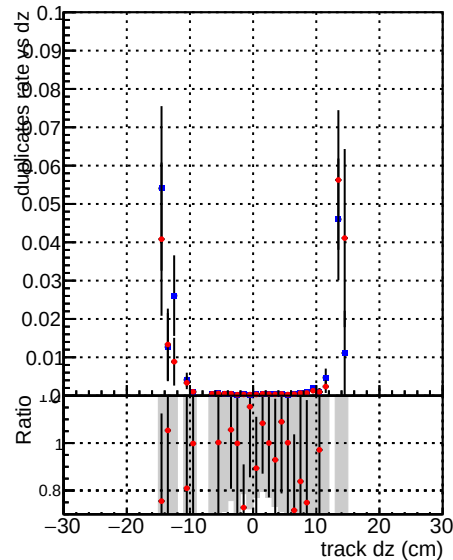
—●— DQM_mkFit5_TTbase —●— DQM_mkFit5_TT_retrainOldFiles125_v2_prelimWP_epoch4
