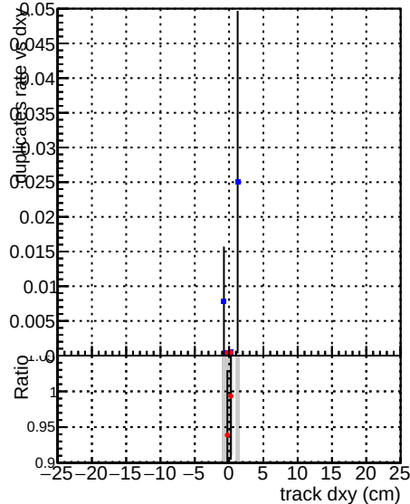
—●— DQM_mkFit5_TTbase —●— DQM_mkFit5_TT_retrainOldFiles125_v2_prelimWP_epoch4
