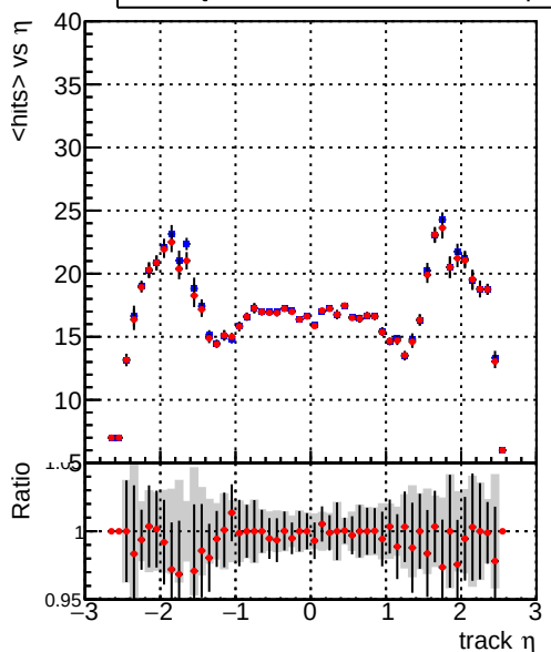
mean hits — DQM_mkFit5_TT_retrainOldFiles125_v2_prelimWP_epoch4
