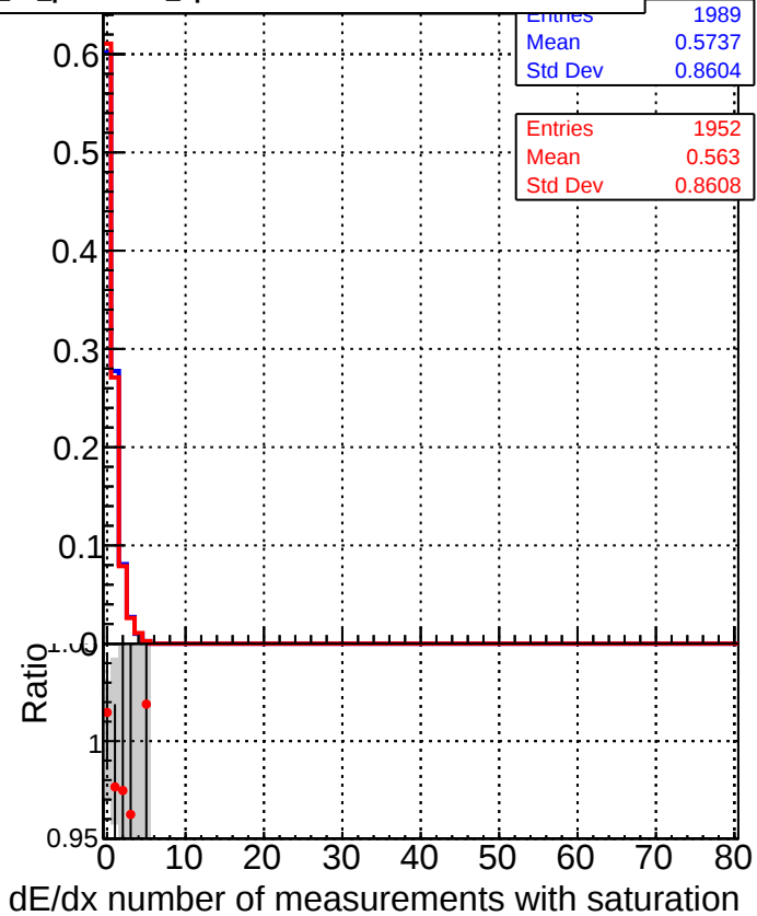
DQM_mkFit_TTbase DQM_mkFit5_TT_retrainOldFiles125_v2_prelimWP_epoch4
