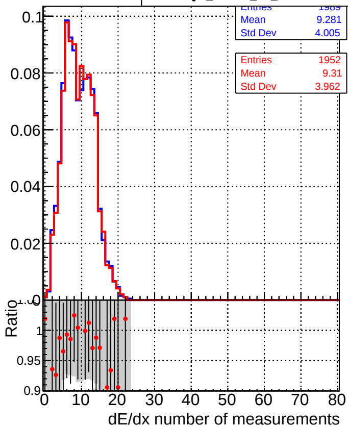
DQM_mkFit_TTbase DQM_mkFit5_TT_retrainOldFiles125_v2_prelimWP_epoch4
