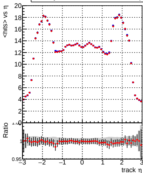
— DQM_mkFit_TTbase — DQM_mkFit5_TT_retrainOldFiles125_v2_prelimWP_epoch4
