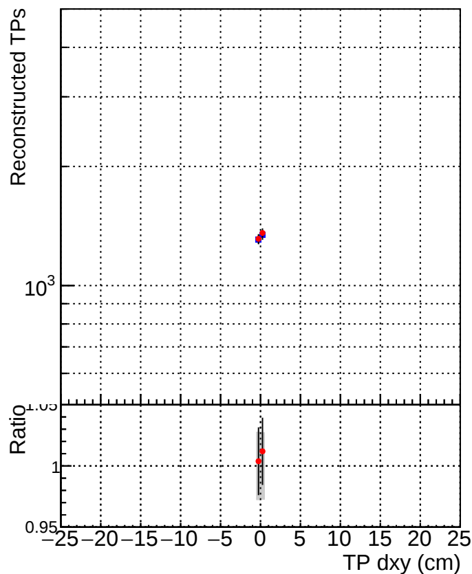
■ DQM_mkFit_TTbase ■ DQM_mkFit5_TT_retrainOldFiles125_v2_prelimWP_epoch4
