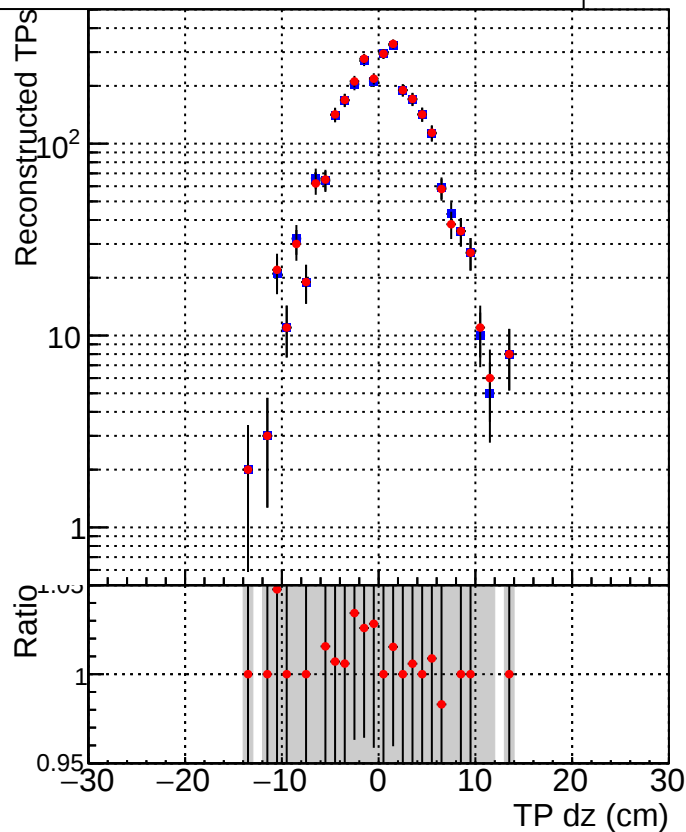
■ DQM_mkFit_TTbase ■ DQM_mkFit5_TT_retrainOldFiles125_v2_prelimWP_epoch4
