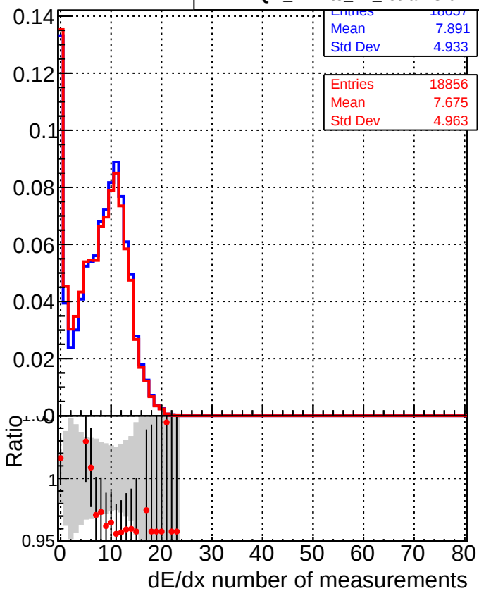
■ DQM_mkFit5_TTbase ● DQM_mkFit5_TT_retrainOldFiles125_v2_prelimWP_epoch4
