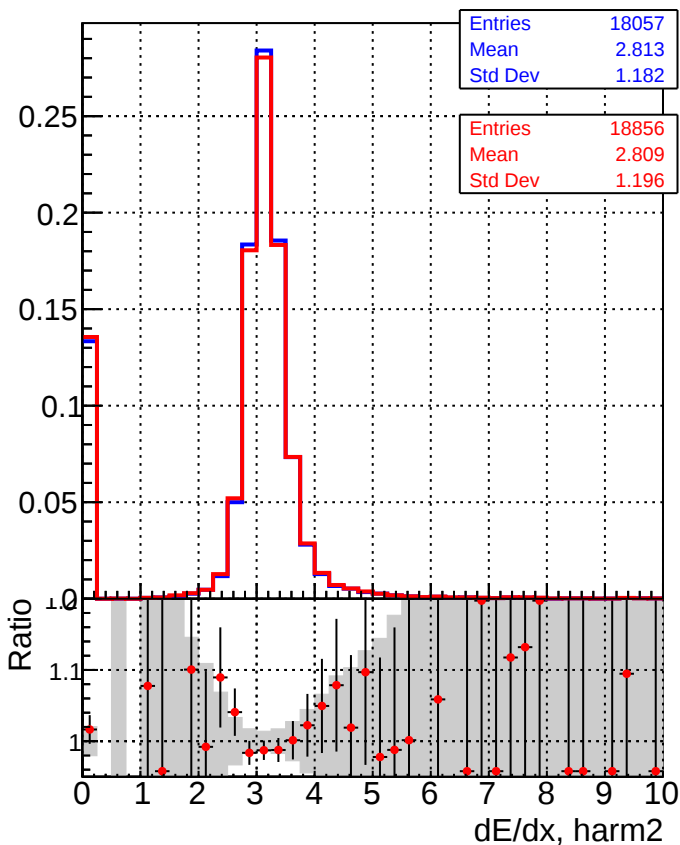
■ DQM_mkFit5_TTbase ● DQM_mkFit5_TT_retrainOldFiles125_v2_prelimWP_epoch4
