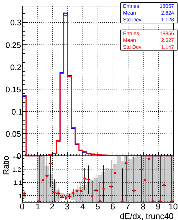
■ DQM_mkFit5_TTbase ● DQM_mkFit5_TT_retrainOldFiles125_v2_prelimWP_epoch4
