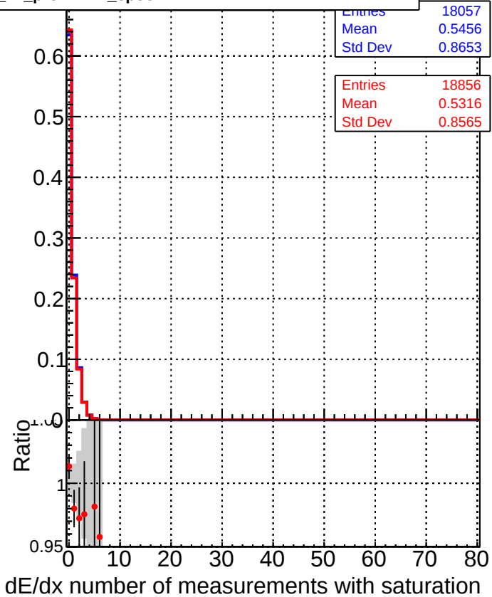
■ DQM_mkFit5_TTbase ● DQM_mkFit5_TT_retrainOldFiles125_v2_prelimWP_epoch4
