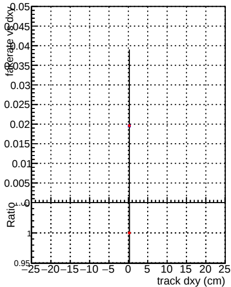
—•— DQM_mkFit_TTbase —•— DQM_mkFit5_TT_retrainOldFiles125_v2_prelimWP_epoch4
