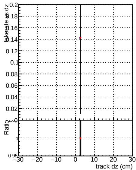
—•— DQM_mkFit_TTbase —•— DQM_mkFit5_TT_retrainOldFiles125_v2_prelimWP_epoch4
