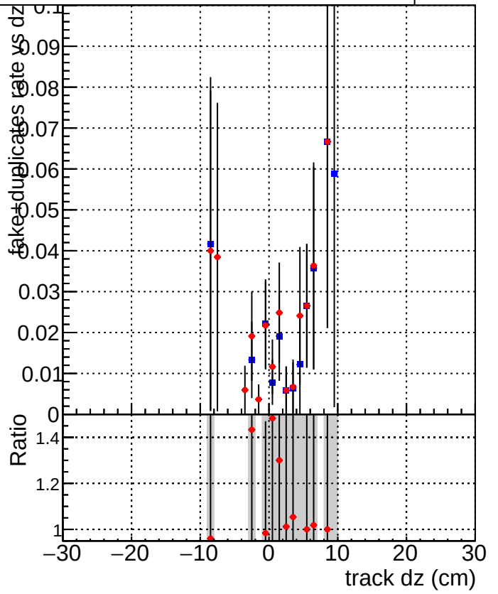
DQM_mkFit_TTbase DQM_mkFit5_TT_retrainOldFiles125_v2_prelimWP_epoch4
