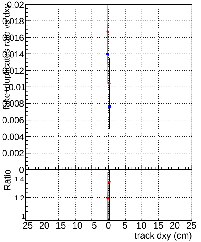
DQM_mkFit_TTbase DQM_mkFit5_TT_retrainOldFiles125_v2_prelimWP_epoch4
