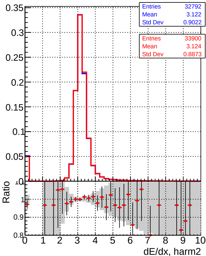
■ DQM_mkFit_TTbase ● DQM_mkFit5_TT_retrainOldFiles125_v2_prelimWP_epoch4
