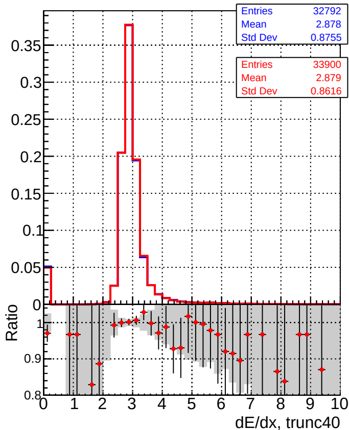
■ DQM_mkFit_TTbase ● DQM_mkFit5_TT_retrainOldFiles125_v2_prelimWP_epoch4
