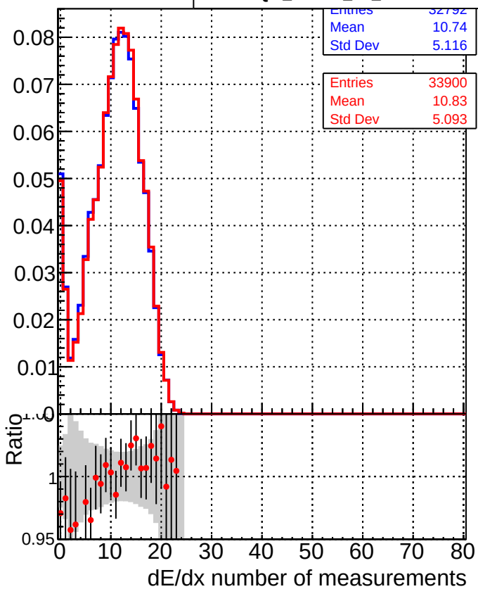
■ DQM_mkFit_TTbase ● DQM_mkFit5_TT_retrainOldFiles125_v2_prelimWP_epoch4
