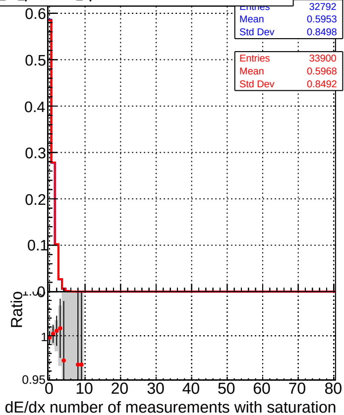
■ DQM_mkFit_TTbase ● DQM_mkFit5_TT_retrainOldFiles125_v2_prelimWP_epoch4
