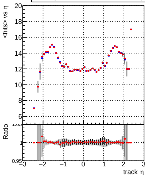
— DQM_mkFit5_TTbase — DQM_mkFit5_TT_retrainOldFiles125_v2_prelimWP_epoch4
