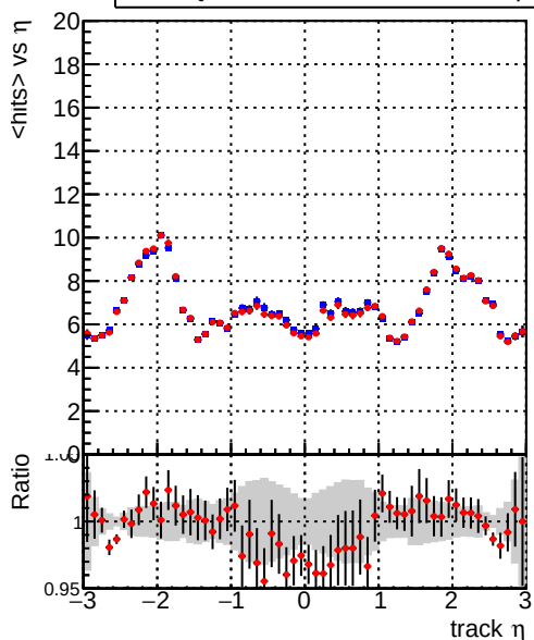
— DQM_mkFit5_TTbase — DQM_mkFit5_TT_retrainOldFiles125_v2_prelimWP_epoch4
