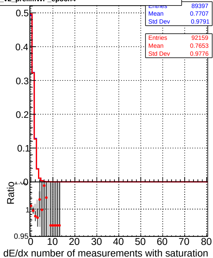
—■— DQM_mkFit_TTbase —●— DQM_mkFit5_TT_retrainOldFiles125_v2_prelimWP_epoch4
