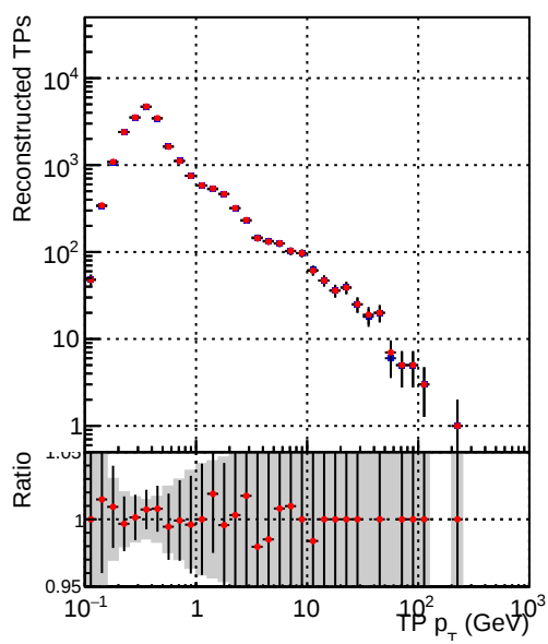
—•— DQM_mkFit_TTbase —•— DQM_mkFit5_TT_retrainOldFiles125_v2_prelimWP_epoch4
