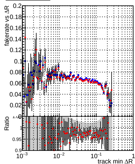
—•— DQM_mkFit_TTbase —•— DQM_mkFit5_TT_retrainOldFiles125_v2_prelimWP_epoch4
