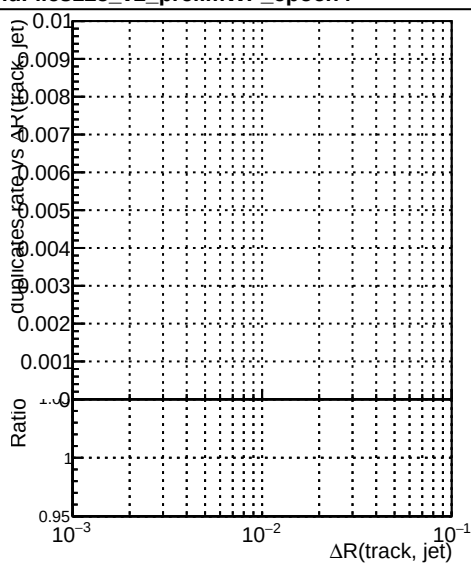
—•— DQM_mkFit_TTbase —•— DQM_mkFit5_TT_retrainOldFiles125_v2_prelimWP_epoch4
