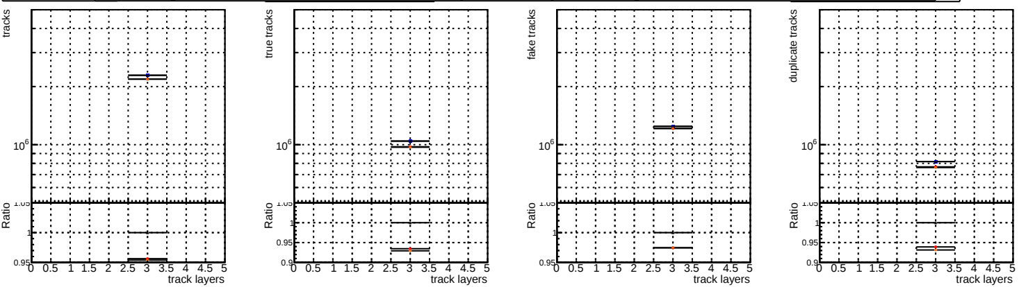
DOM mkIt5 TTbase DOM mkIt5 TTretrainOldFiles125 v2 prelimWP epoch4 DOM mkIt6 TTbaseline_6iter DOM mkIt6 TTretrainOldFiles125 v2 prelimWP epoch2 wSQCD
