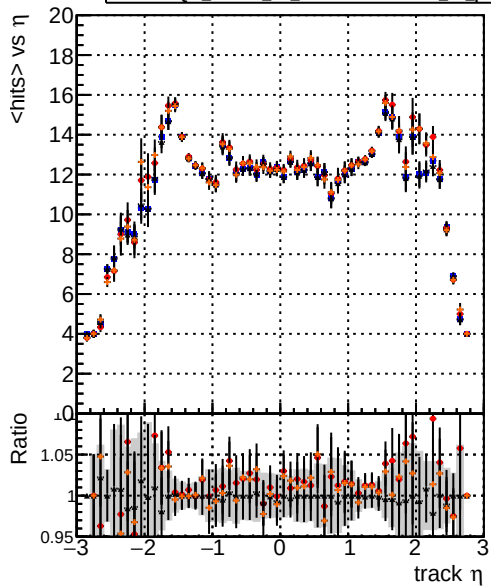
mean hits DQM_mkFit1_TTbase DQM_mkFit5_TT_retrainOldFiles125_v2_prelimWP_epoch4 DQM_mkFit6_TT_baseLine_6iter DQM_mkFit6_TT_retrainOldFiles125_v2_prelimWP_epoch2_wsQCD
