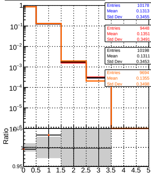
mean hits DQM_mkFit1_TTbase DQM_mkFit5_TT_retrainOldFiles125_v2_prelimWP_epoch4 DQM_mkFit6_TT_baseLine_6iter DQM_mkFit6_TT_retrainOldFiles125_v2_prelimWP_epoch2_wsQCD
