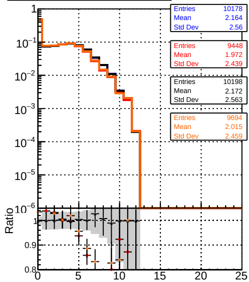
mean hits DQM_mkFit1_TTbase DQM_mkFit5_TT_retrainOldFiles125_v2_prelimWP_epoch4 DQM_mkFit6_TT_baseLine_6iter DQM_mkFit6_TT_retrainOldFiles125_v2_prelimWP_epoch2_wsQCD
