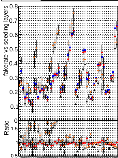
Fake rate vs. ◆ DQM mkFit5 TTbase ■ DQM mkFit5 TTbase ▲ DQM mkFit6 TTbase ◆ DQM mkFit5 TTbase ■ DQM mkFit5 TTbase ▲ DQM mkFit6 TTbase ◆ DQM mkFit5 TTbase ■ DQM mkFit5 TTbase ▲ DQM mkFit6 TTbase ◆ DQM mkFit5 TTbase ■ DQM mkFit5 TTbase ▲ DQM mkFit6 TTbase ◆ DQM mkFit5 TTbase ■ DQM mkFit5 TTbase ▲ DQM mkFit6 TTbase
