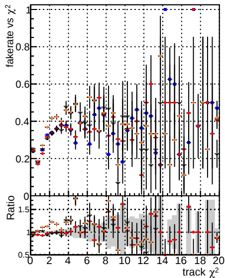
Fake rate vs. ◆ DQM mkFit5 TTbase ■ DQM mkFit5 TTbase ▲ DQM mkFit6 TTbase ◆ DQM mkFit5 TTbase ■ DQM mkFit5 TTbase ▲ DQM mkFit6 TTbase ◆ DQM mkFit5 TTbase ■ DQM mkFit5 TTbase ▲ DQM mkFit6 TTbase ◆ DQM mkFit5 TTbase ■ DQM mkFit5 TTbase ▲ DQM mkFit6 TTbase ◆ DQM mkFit5 TTbase ■ DQM mkFit5 TTbase ▲ DQM mkFit6 TTbase
